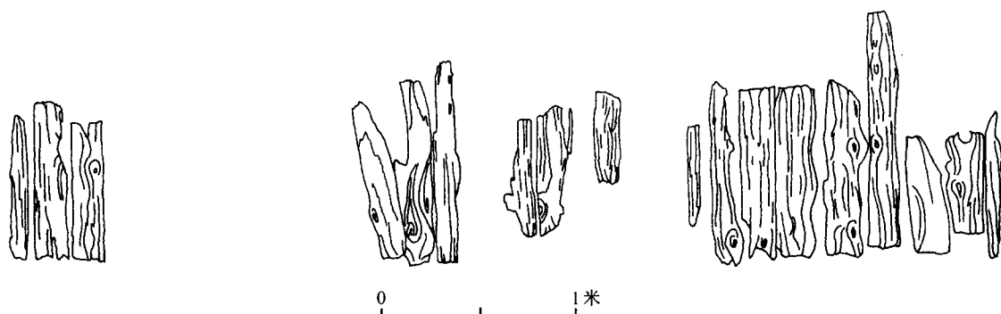
图三 99DRNM1 封土外围柏木圈之一部分（探沟内）
