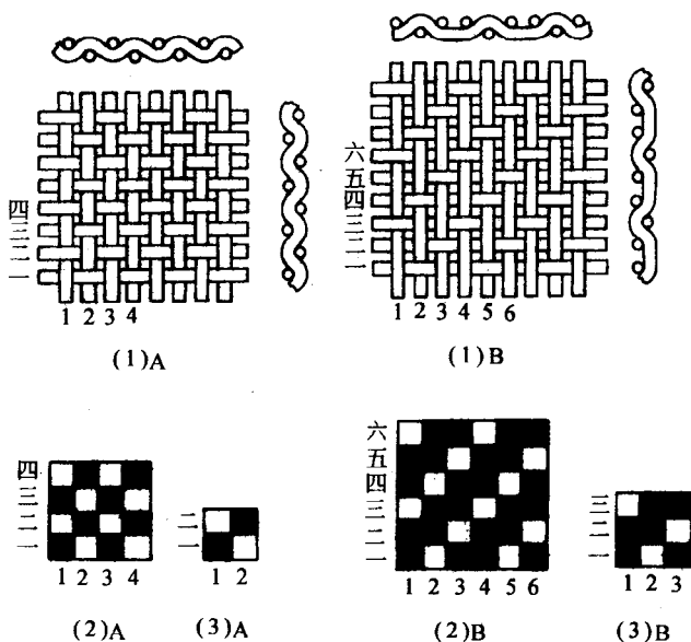
图 1-2 织物的交织片段及其组织图、组织循环
