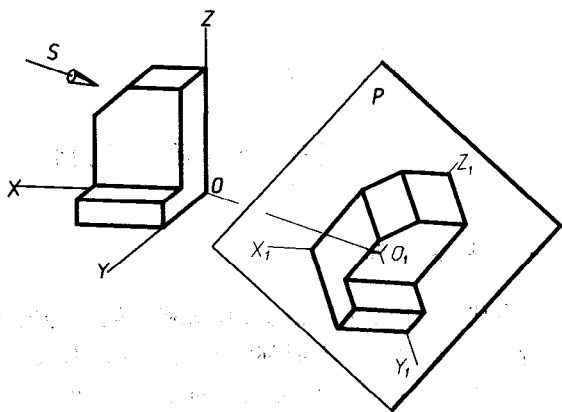
图 0-5 轴测投影法
