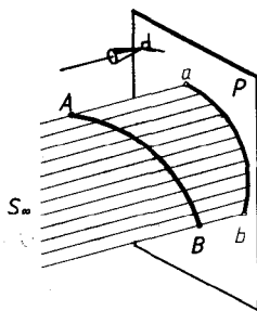
(b) 正投影法
