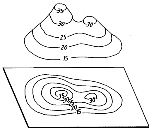
图 0-7 标高投影法
