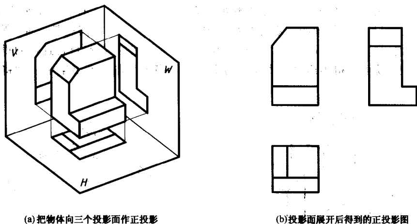
图 0-4 多面正投影法
