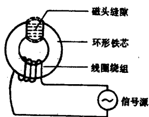
图 1.1.1 视频磁头结构
