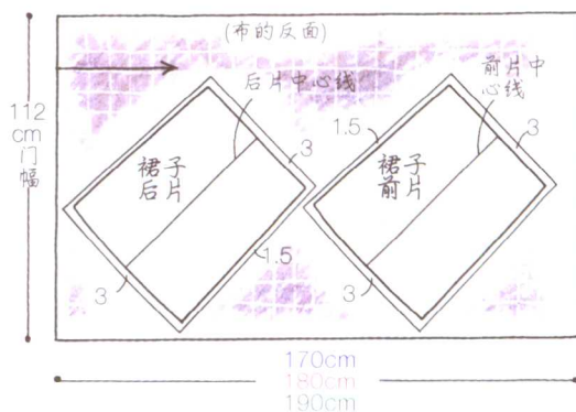
裙布的裁剪图
