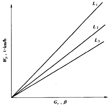
图 1-3 汽车运输生产率 W_p 与汽车载质量 G_c 和行程利用率 \beta 的关系 ( L 为货物运距, 且 L_1 < L_2 < L_3 )
