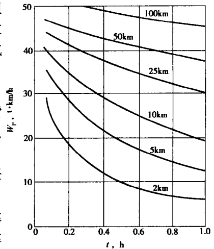
图 1-4 载质量 4t 货车运输生产率 W_p 与车辆每运次装卸货物停歇时间 t 的关系 ( L —运距)
