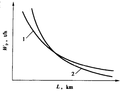
图 1-5 不同车辆的运输生产率 W_p (普通汽车与自卸汽车) 1-普通车辆;2-自装卸车辆
