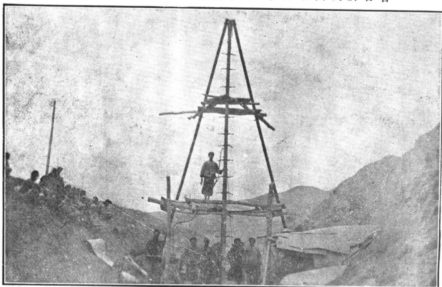
甘肅會靜所屬石界鋪子峽煤礦鑽機全圖 著者於民國十八年冬在甘肅會寧兩縣所屬石界鋪地方煤礦情形攝影
