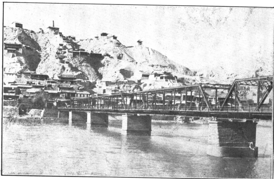
甘肅省蘭縣黃河鐵橋攝影名天下第一橋爲清陝甘總督所建遺
