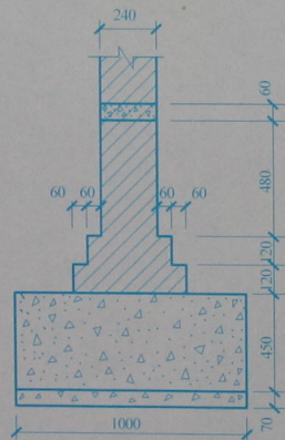
砖墙基础 1:20
