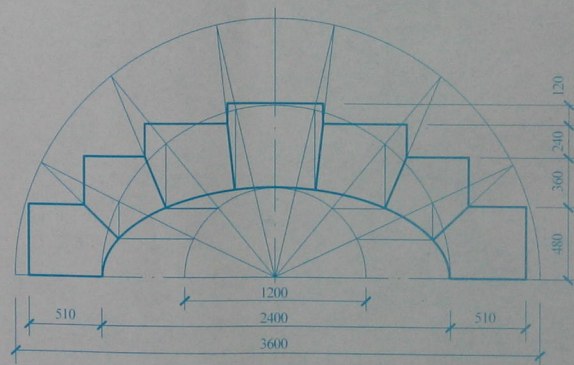
拱门 1:30
