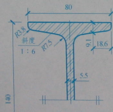
工字钢 1:1
