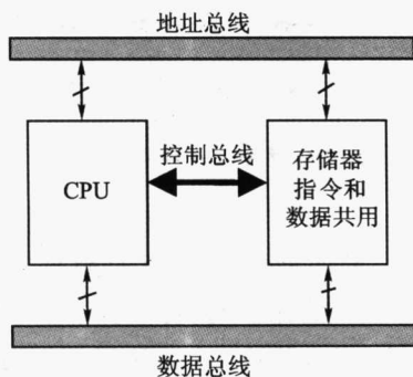
图 1-3 冯·诺依曼(Von-Neumann)结构
