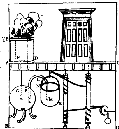
图 1 “庙门自开”的原理
