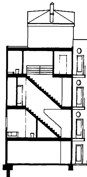
剖面图
