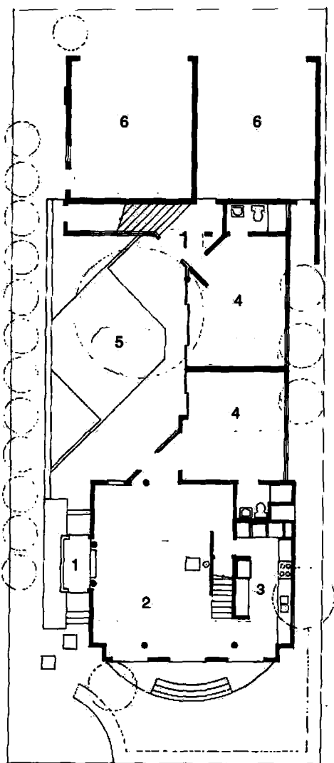
一层平面图/总平面图
