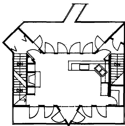
二层平面图
