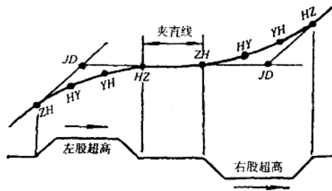
图 1-7 反向曲线示意图
