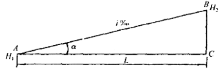
图 1-8 坡道坡度
