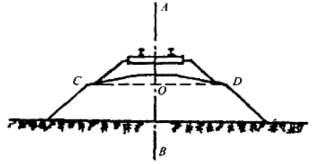
图 1-3 线路中心线位置
