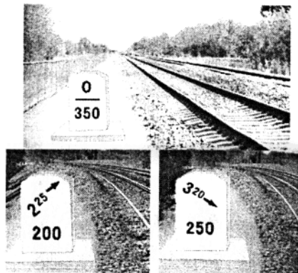
图 1-16 坡度标
