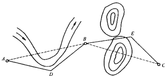
图 1-2 铁路线路绕避地形障碍示意图
