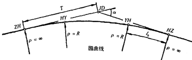
图 1-5 缓和曲线
