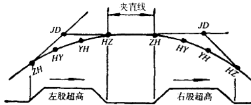
图 1-6 同向曲线示意图
