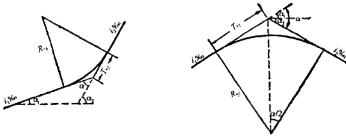
图 1-11 竖曲线的形状
