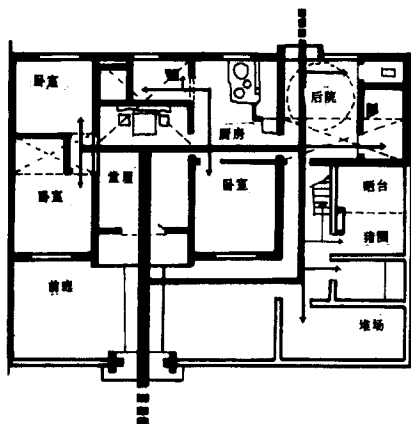
南方农民平房住宅平面
