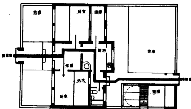
北方农民平房住宅平面
