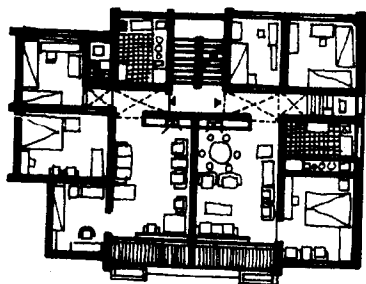
梯间式平面
