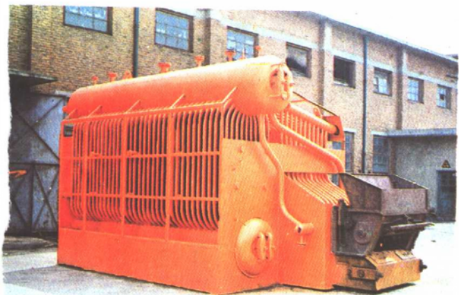
该厂生产的S2L4-13-A II水管快装蒸汽锅炉
