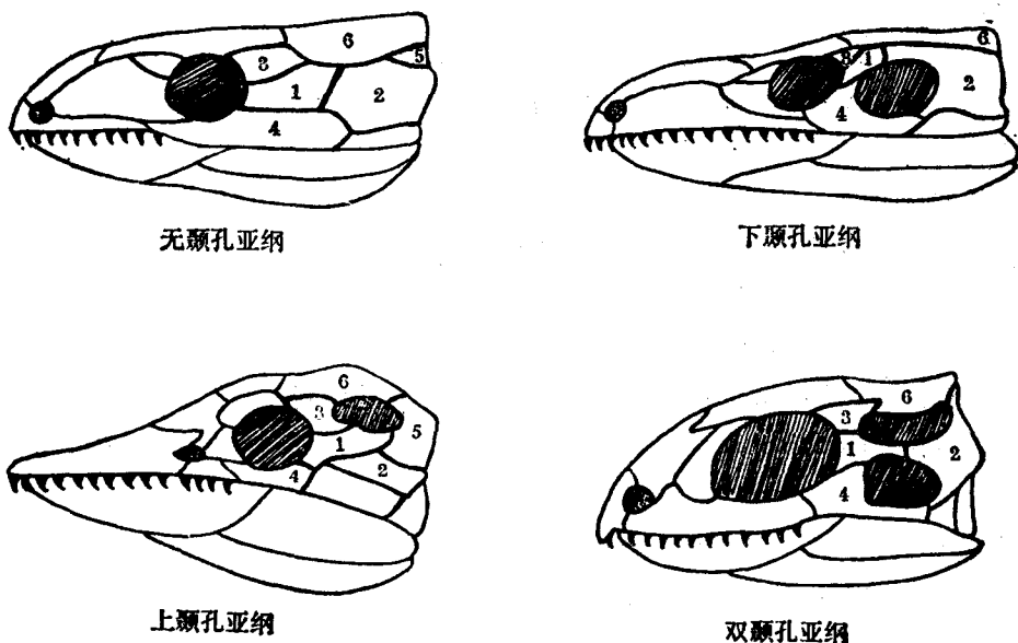
图1 爬行类四亚纲头骨示意图
