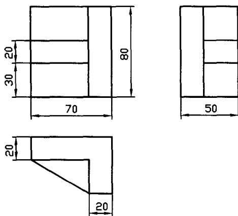
图 2-4 三视图 1
