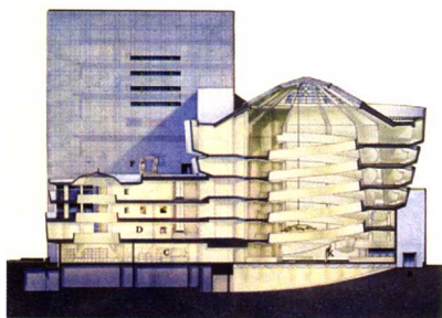
圆形大厅剖面图
