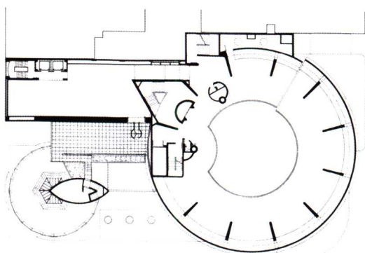
六层平面图
