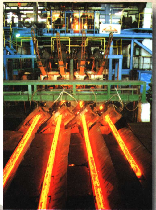
方坯连铸机
