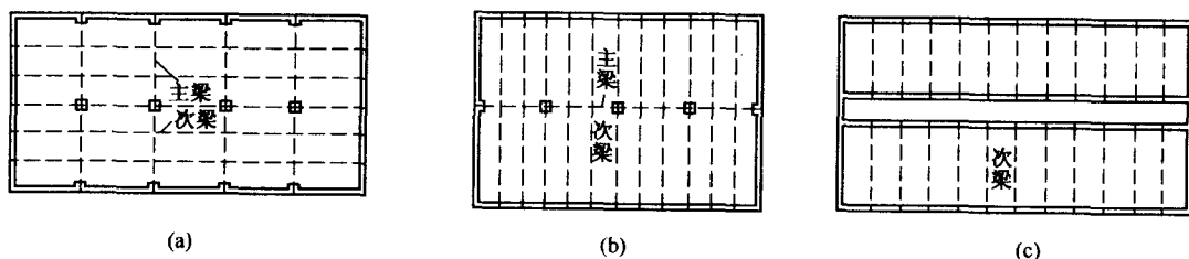
图 1—5 梁格布置
