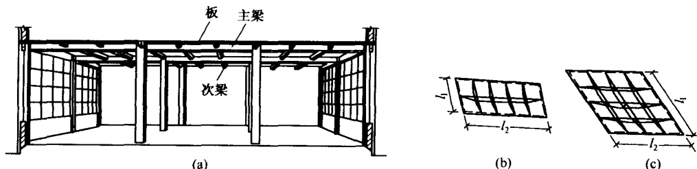
图 1-1 肋梁楼盖
