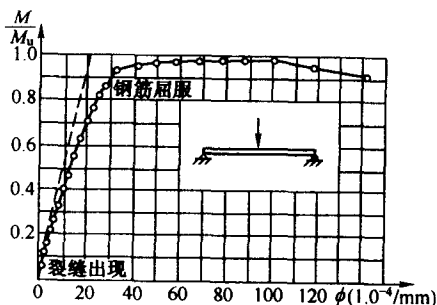
图1—11 实测 M - \phi 关系曲线
