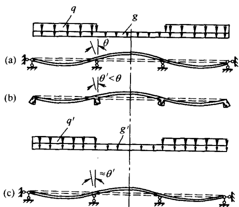
图1—7 折算荷载
