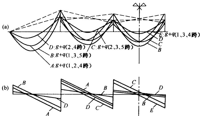
图1—9 内力包络图 (a)弯矩包络图;(b)剪力包络图。
