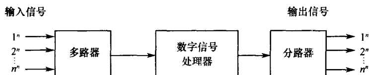
图1-1 时分复用系统
