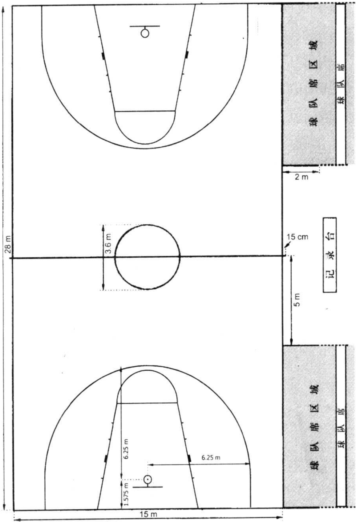
图 1 球场的全部尺寸
