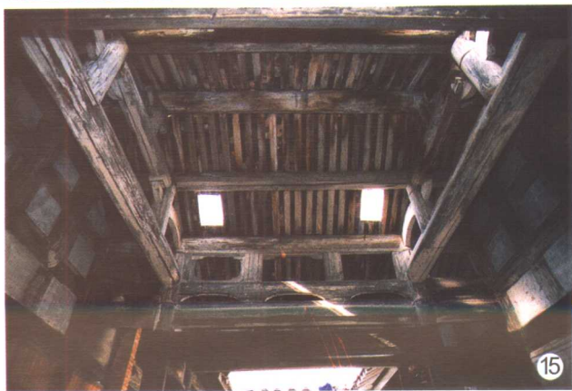
大宗伯第厅堂梁架结构 全貌
