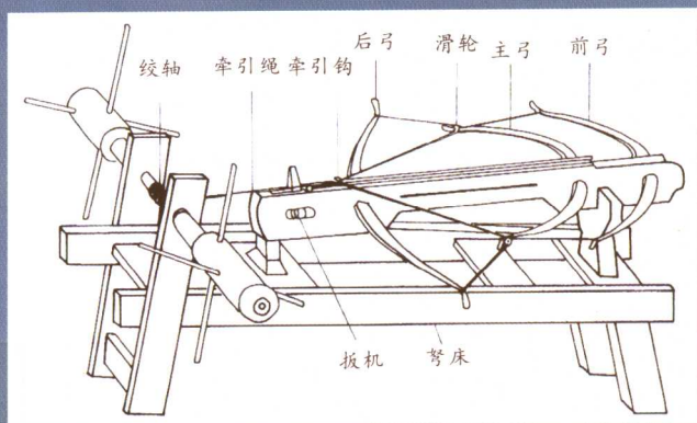
三弓床弩示意图。
