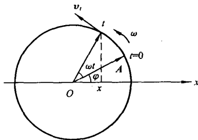
图 13.1.7 旋转矢量与简谐振动
