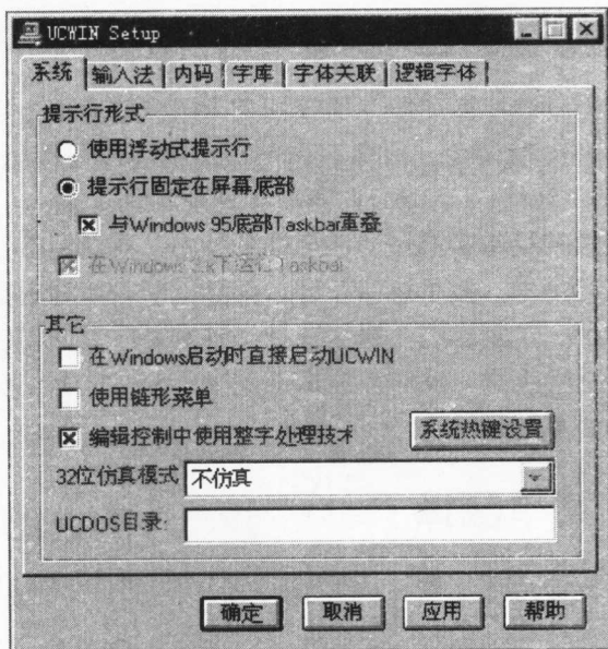
图 3-5 UCWIN 的系统设置对话框
