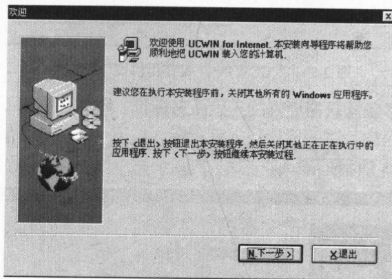
图 2-1 “欢迎”窗口
