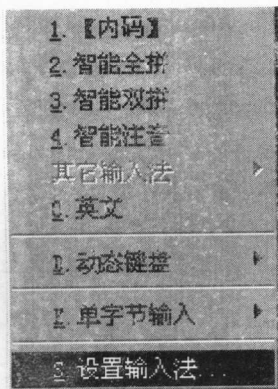
图 3-3 输入法菜单
