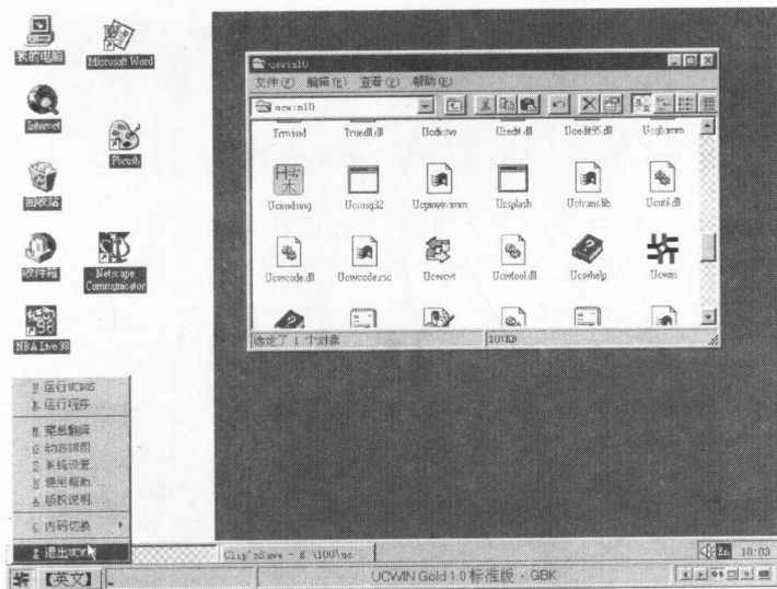
图 3-1 启动 UCWIN
