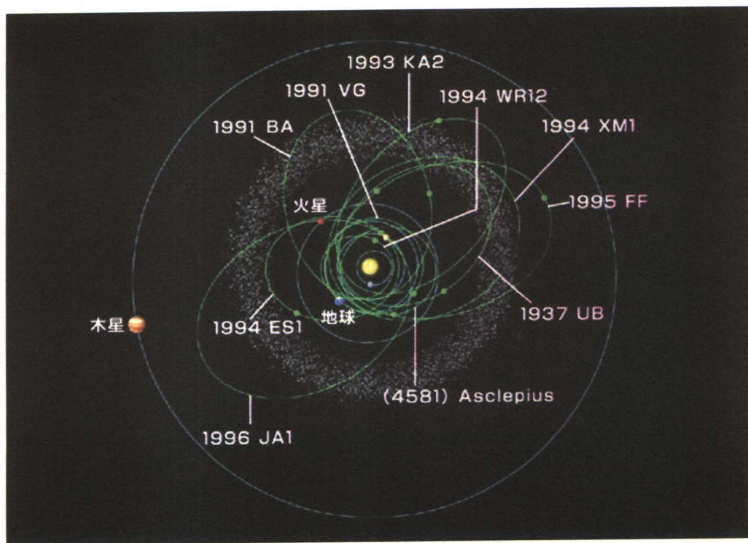
有的小行星的轨道非常接近地球，图中画出了10颗这样的小行星：1996JA1、1994ES1、1991BA、1991VG、1993KA2、1994WR12、1994XM1、1995FF、1937UB和（4581）Asclepius
