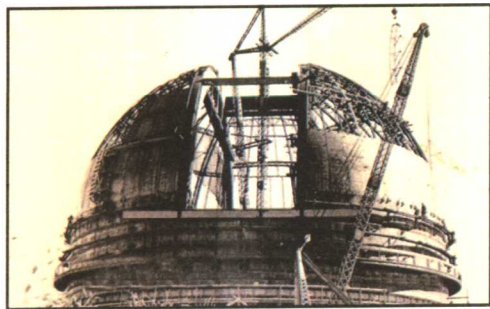
20世纪初，帕洛玛山天文台5.08米望远镜开始修建，它曾经是世界上最大口径的望远镜。在研究天文学的基本问题，如星系的形成与演化、宇宙的年龄和构造，寻找类星体等方面，这台望远镜发挥了巨大的作用
