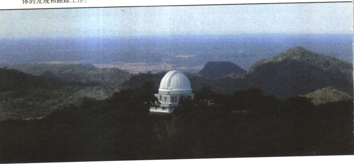
澳大利亚AAO天文台
