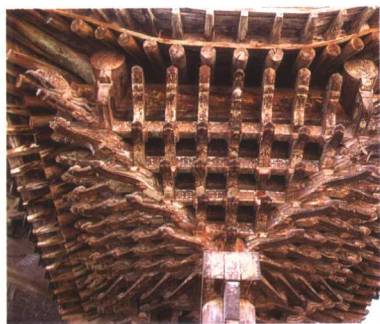
太谷县阳邑镇净信寺戏台八字墙斗拱
