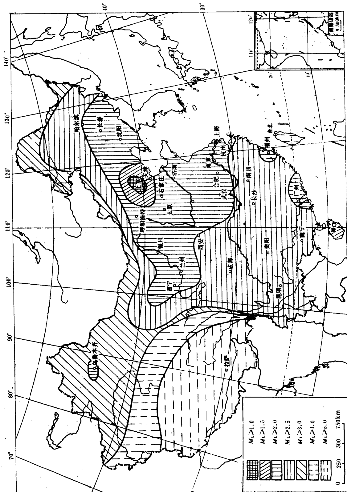
中国区域地震台网监测能力略图 (1982年)
