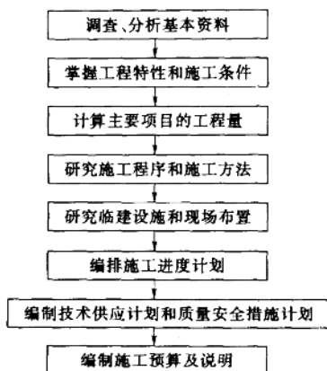
图 1-2 施工组织设计编制步骤程序图
