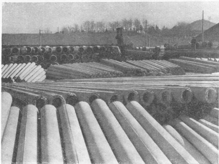
烟台水泥制品厂利用当地生产的水泥，加工成水泥管、电线杆，支援农村水利、电力建设。
