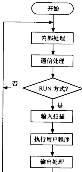
图 1-1 工作原理图
