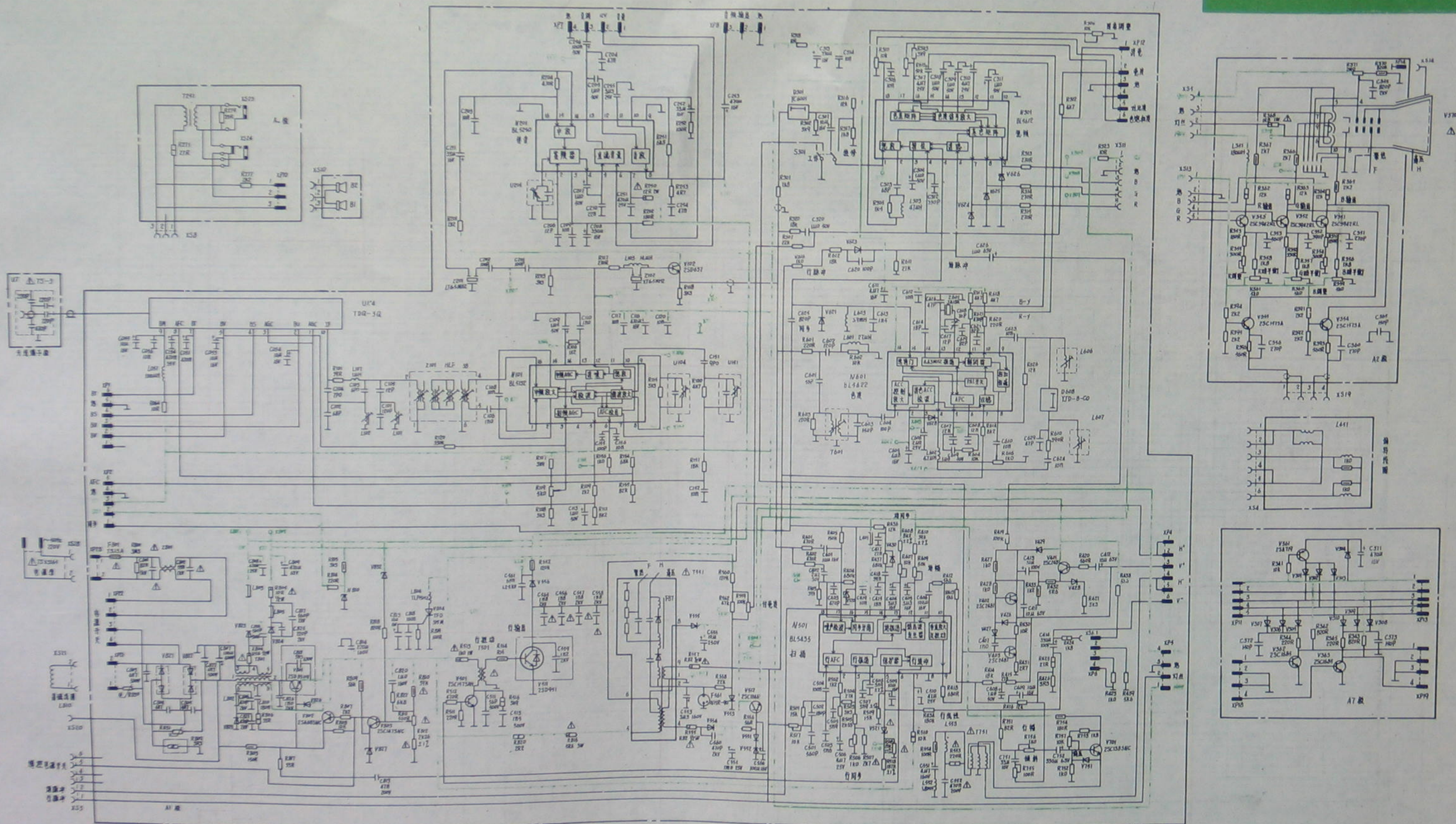
47CD3/SR5105 彩色电视接收机电路图 (主机线路)
