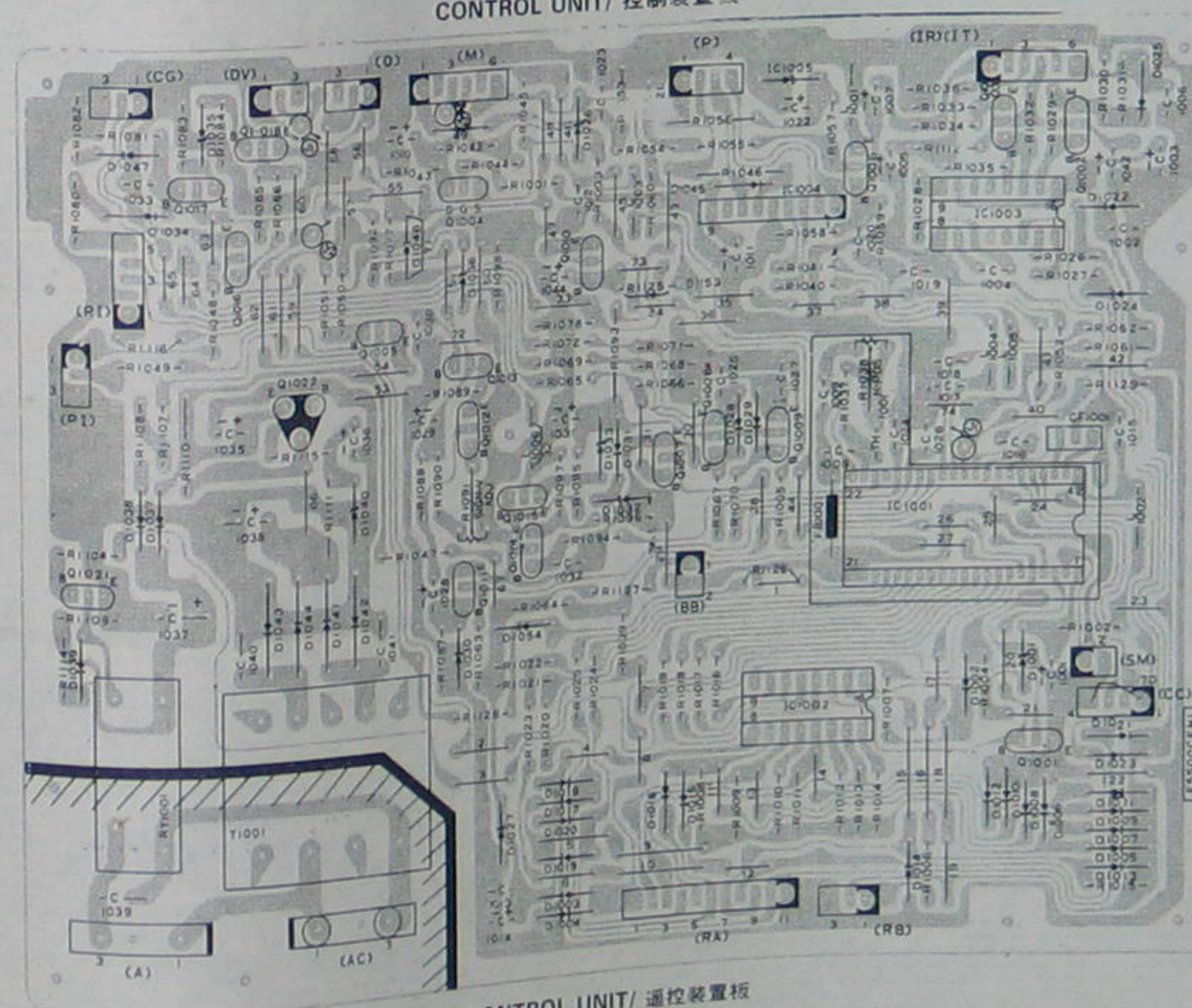
印制电路板图
