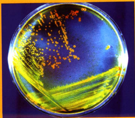
可以承受高强度辐射的恐兽球菌（黄色），它只能生长在琼脂培养基里，科学家推测其来自火星
