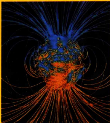
科学家发现地球磁场南北 翻转有前兆
