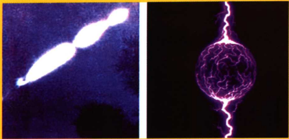
神秘的球状闪电
