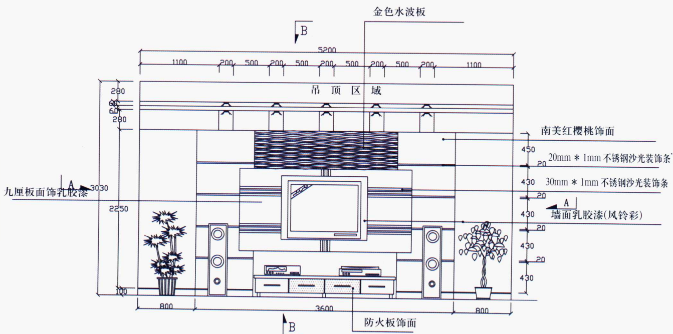
电视背景墙立面图 S1:100
