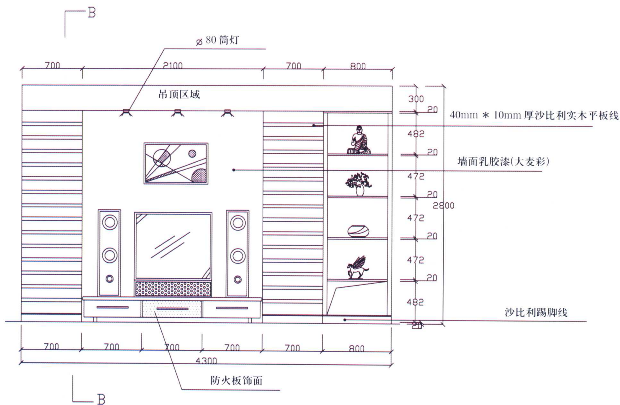
电视背景墙立面图 S1:100
