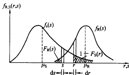
图 1-1-1 R 和 S 的密度函数与失效概率
