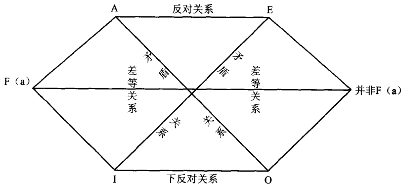
图 1-7 对当方阵
