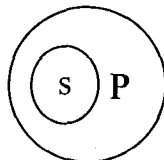
图 1-2 真包含关系与真包含关系欧拉图
