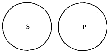
图 1-4 全异关系欧拉图
