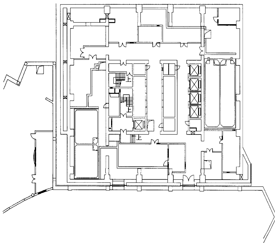
一号主楼地下层平面图
