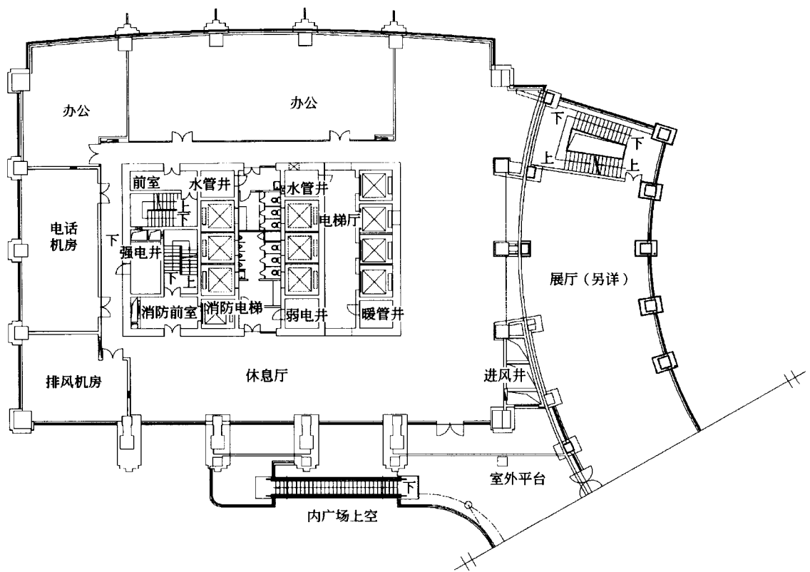
复兴大厦二号楼三层平面图
