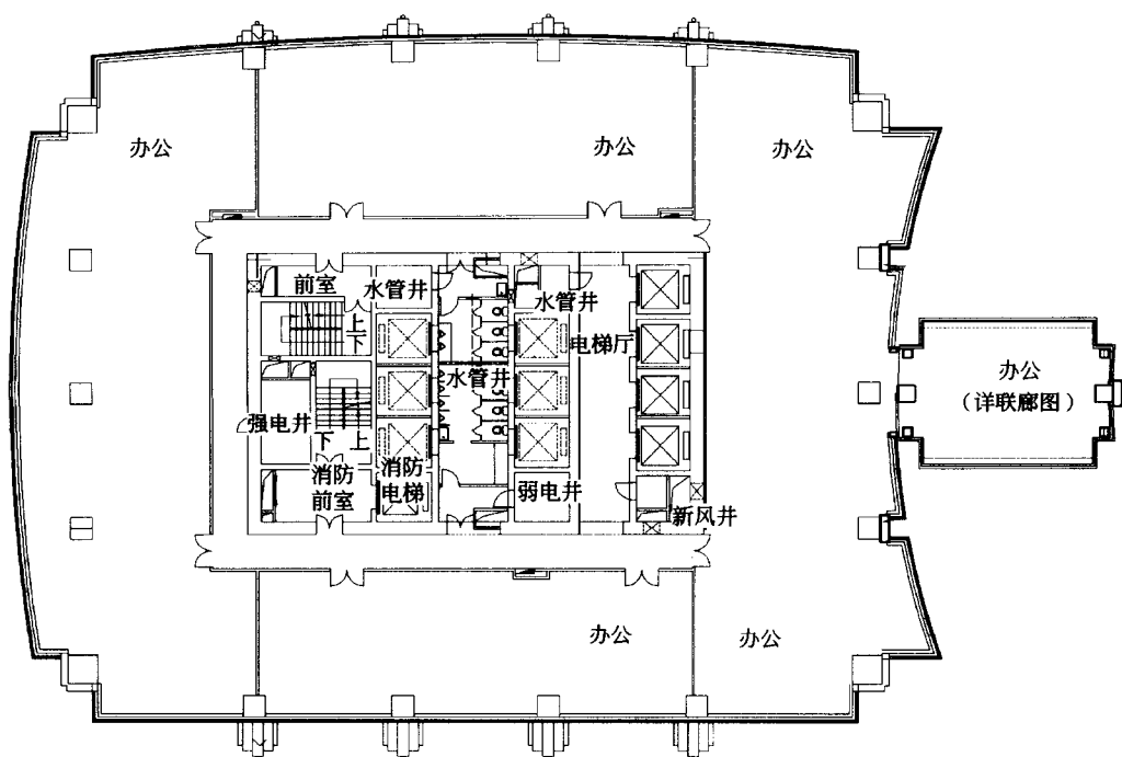
复兴大厦二号楼八、九层平面图
