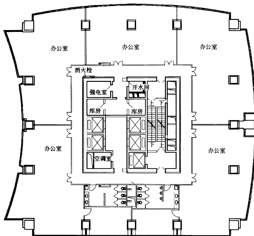
一号主楼三十三层平面图
