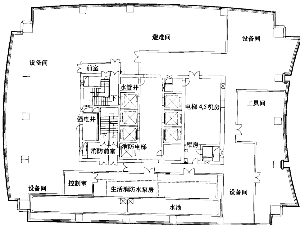
复兴大厦二号楼十五和三十(避难)层平面图
