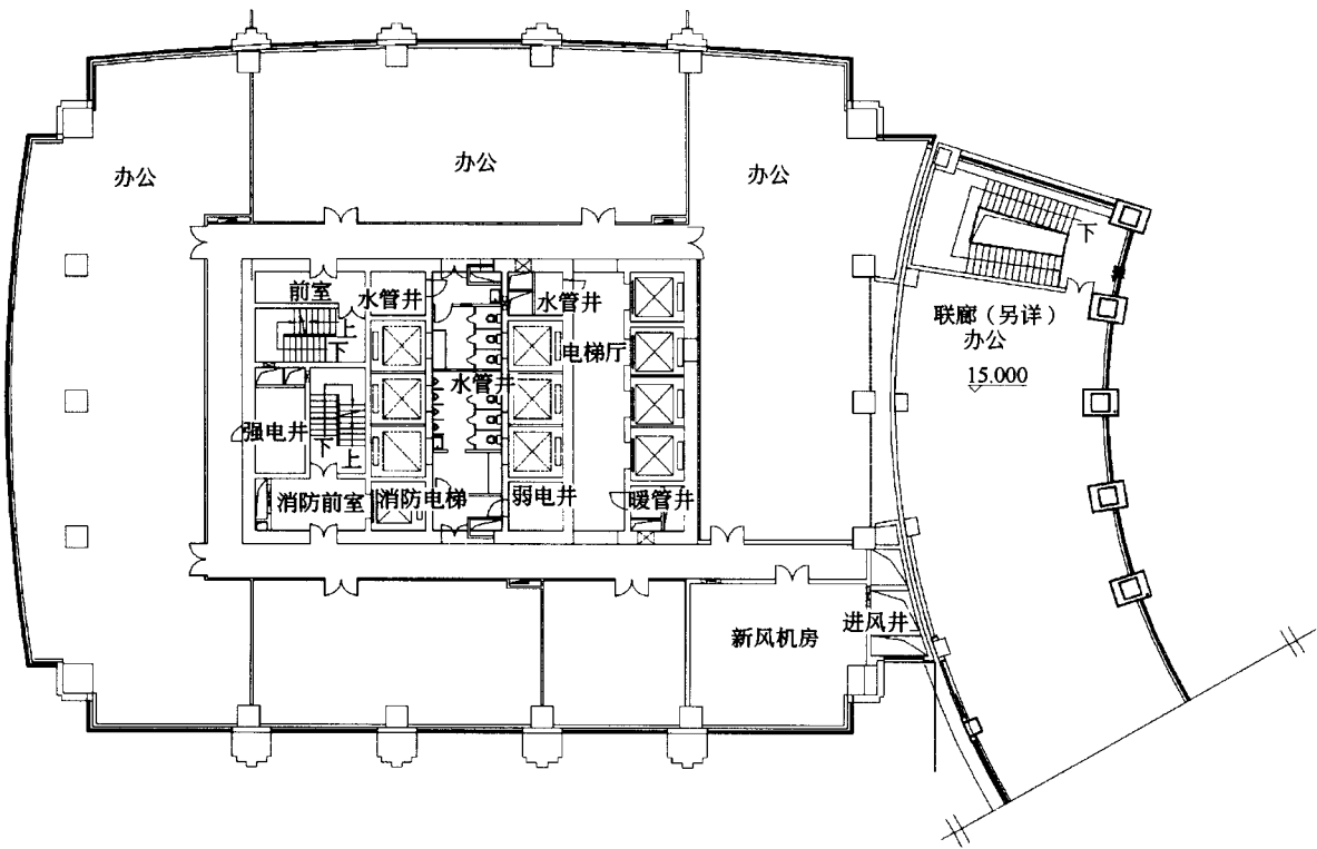
复兴大厦二号楼四层平面图
