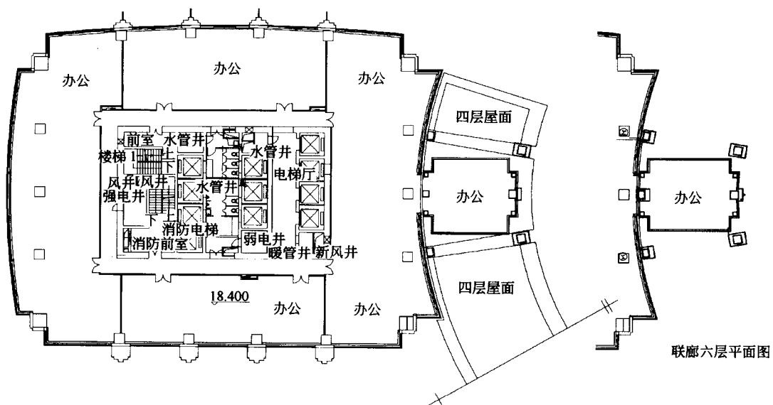
复兴大厦二号楼五、六层平面图
