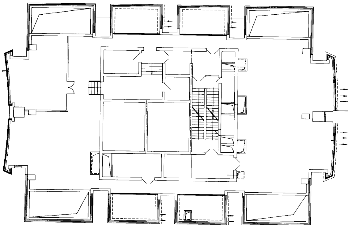
一号主楼四十一层平面图
