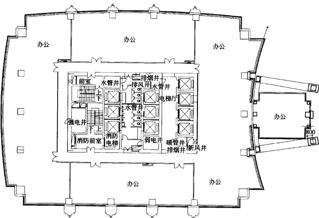
复兴大厦二号楼七层平面图
