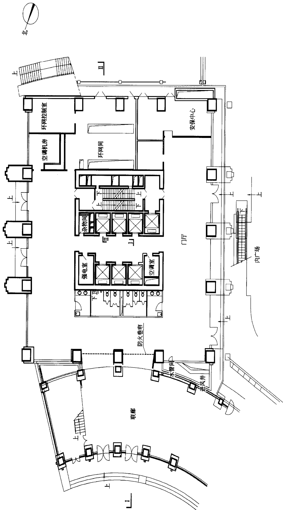
一号主楼一层平面图
