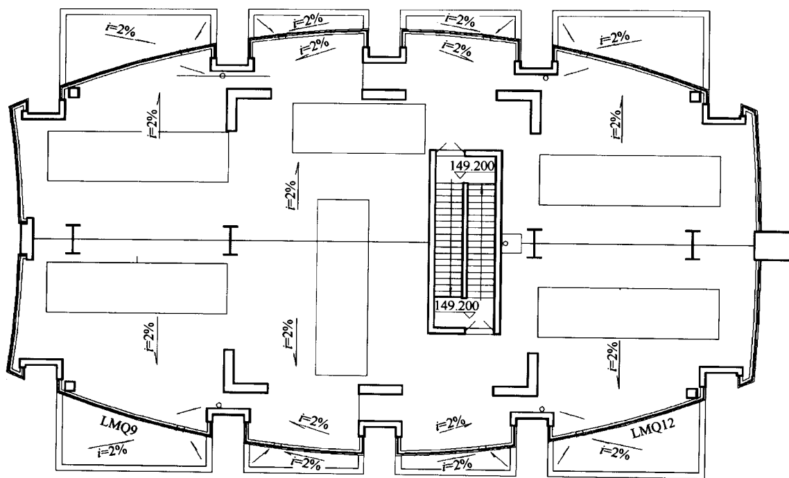
一号主楼屋顶平面图
