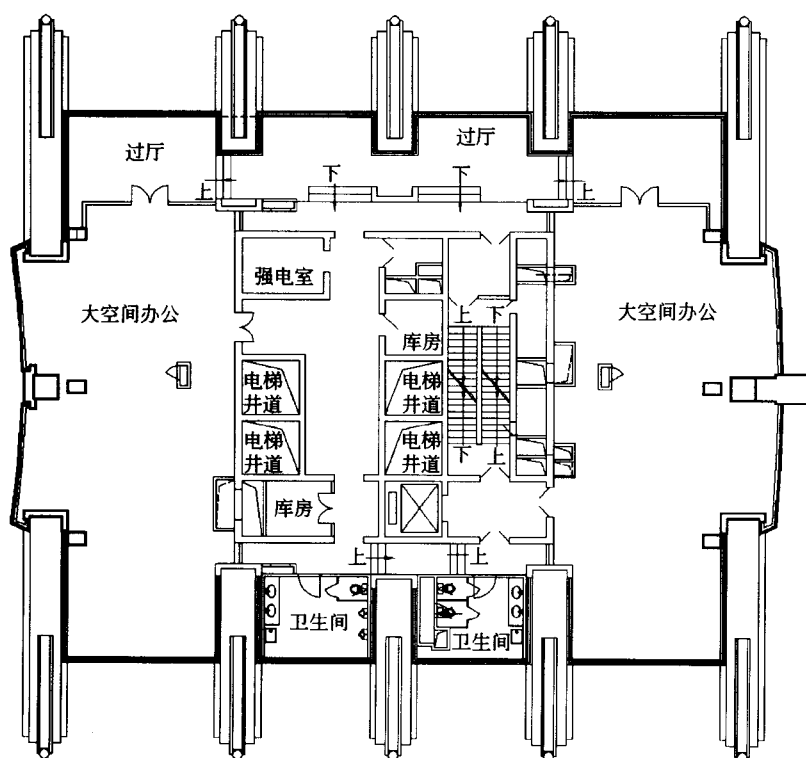
一号主楼四十层平面图
