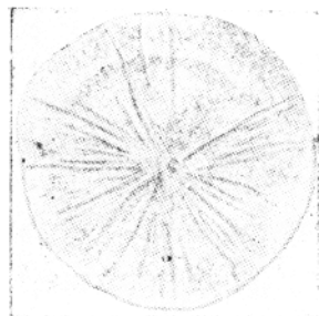
圖7 結核
