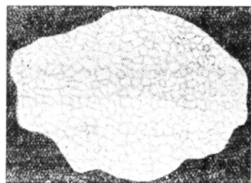
圖8 鮑狀結構
