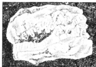
圖10 晶洞
