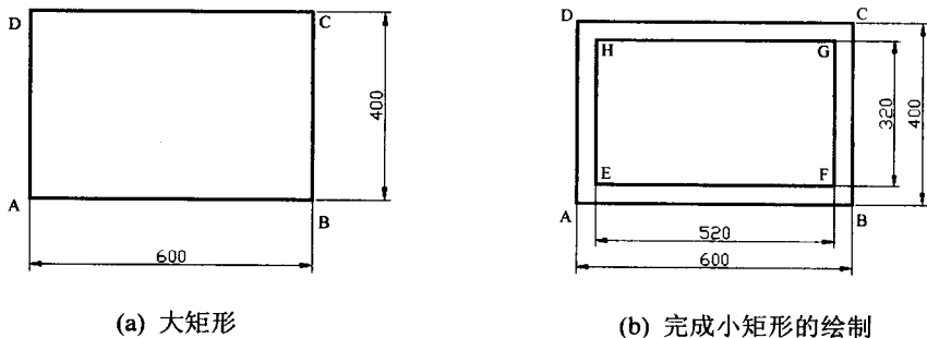
图 1-21 绘制小矩形
