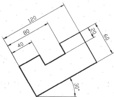
图 1-6 倾斜水槽
