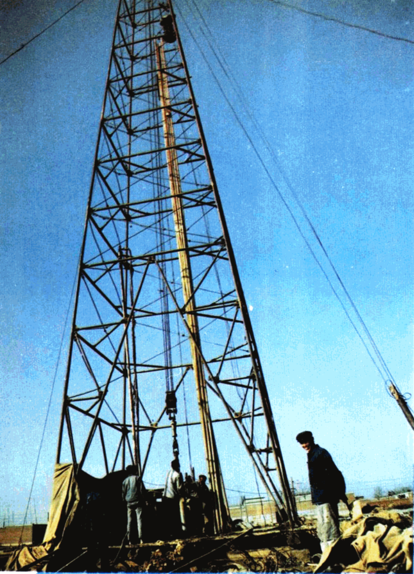
机井建设
