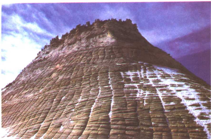
在美国宰恩国家公园中，红色砂岩被风和雨雕凿成棋盘状形状
