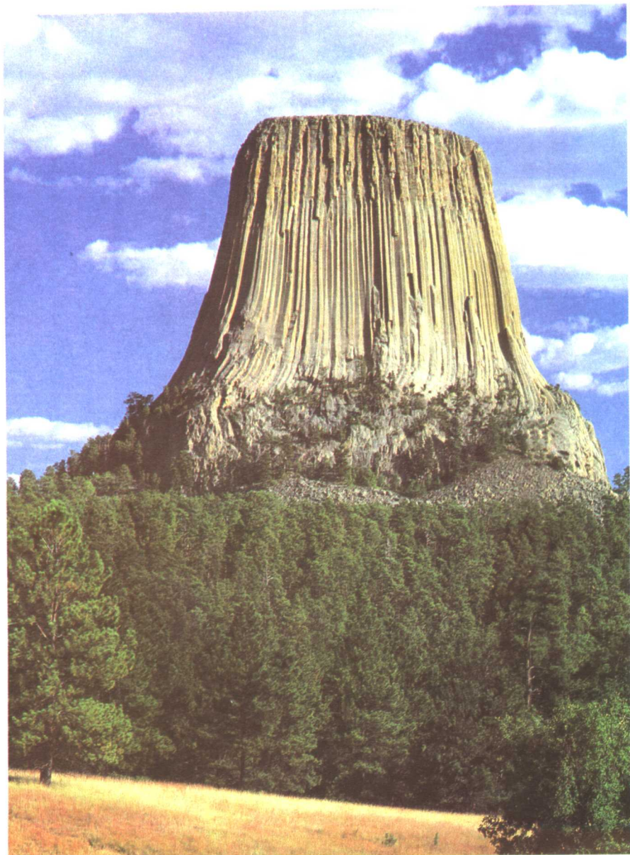
屹立于美国怀俄明州东北部平原上的魔鬼塔，它的巨型柱状熔岩构造形成于5000万年前
