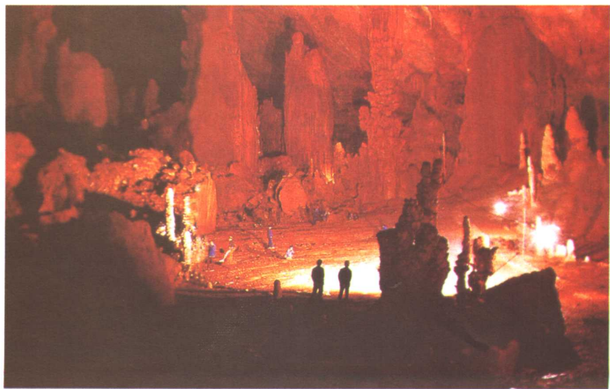
这是贵州省发现的一个长350米、宽170米、高50米的巨型地底溶洞厅，洞中耸立着石笋林，洞内还有清澈的间隙泉。
