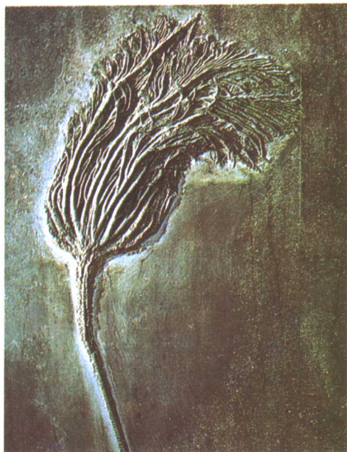
古代芦木叶化石
