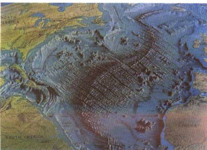
大西洋海底地貌图
