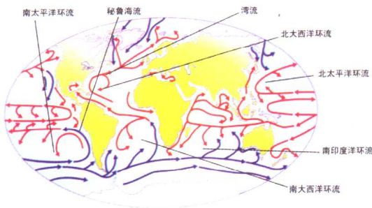
海流示意图
