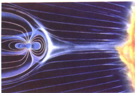
地球磁场
