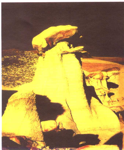
新疆雅丹地貌
