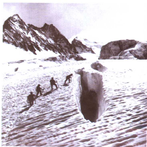
冰川
