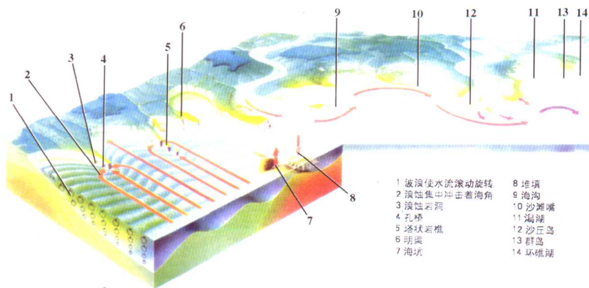
海洋构造图
