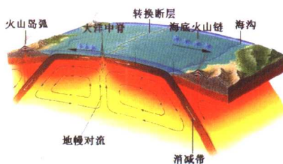
板块构造
