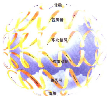
信风图
