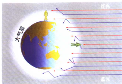
地球的光照
