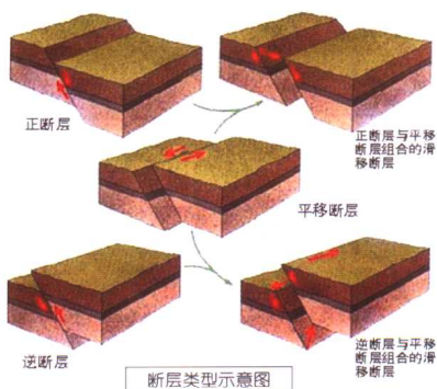
断层类型示意图
