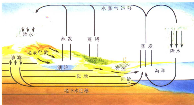
水气循环
