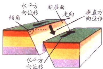
断层位移示意图
