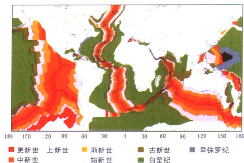
海盆的年龄
