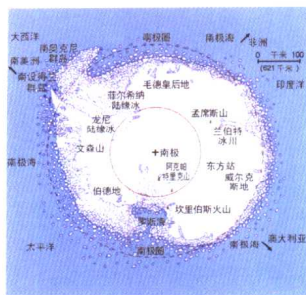
南极地图
