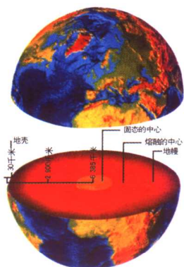
地球的内部构造
