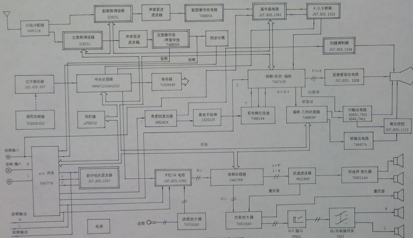
长虹 C2518 系列整机电路方框图
