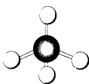
(a) 棍球模型
