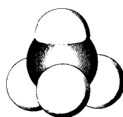
(b) 比例模型
