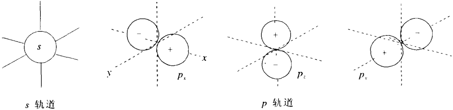
图 1-3 原子轨道
