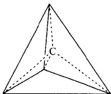
图 1-1 碳原子的四面体模型
