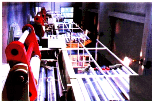
从意大利引进的PVC抗皱包装膜生产线
