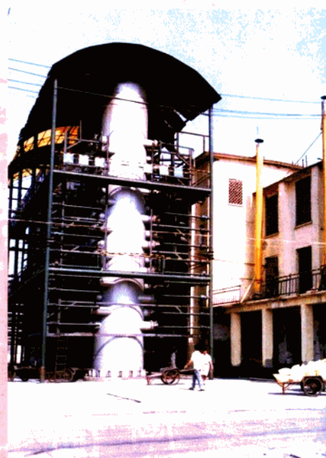
碳化塔
