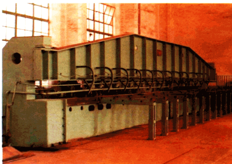
大型刨边机
