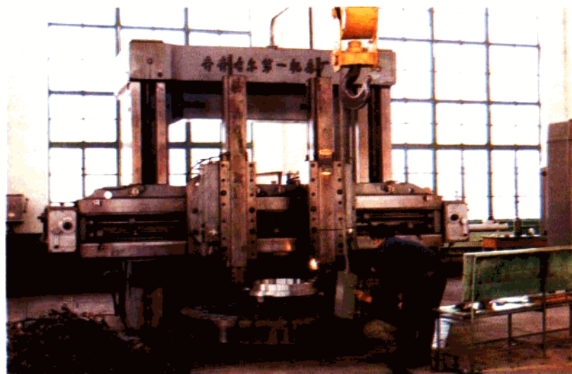
直径2.5米的立式车床
