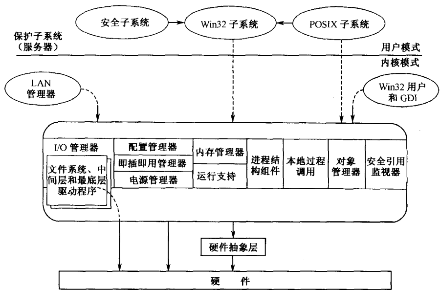
图 1-1 Windows 2000 组件总览
