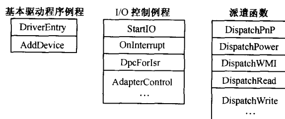
图 1-3 WDM 驱动程序例程
