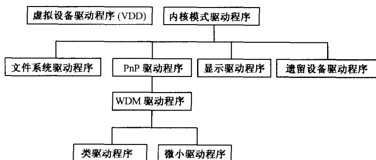
图 1-2 Windows 2000 中的设备驱动程序种类
