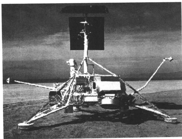
“勘探者”3号
