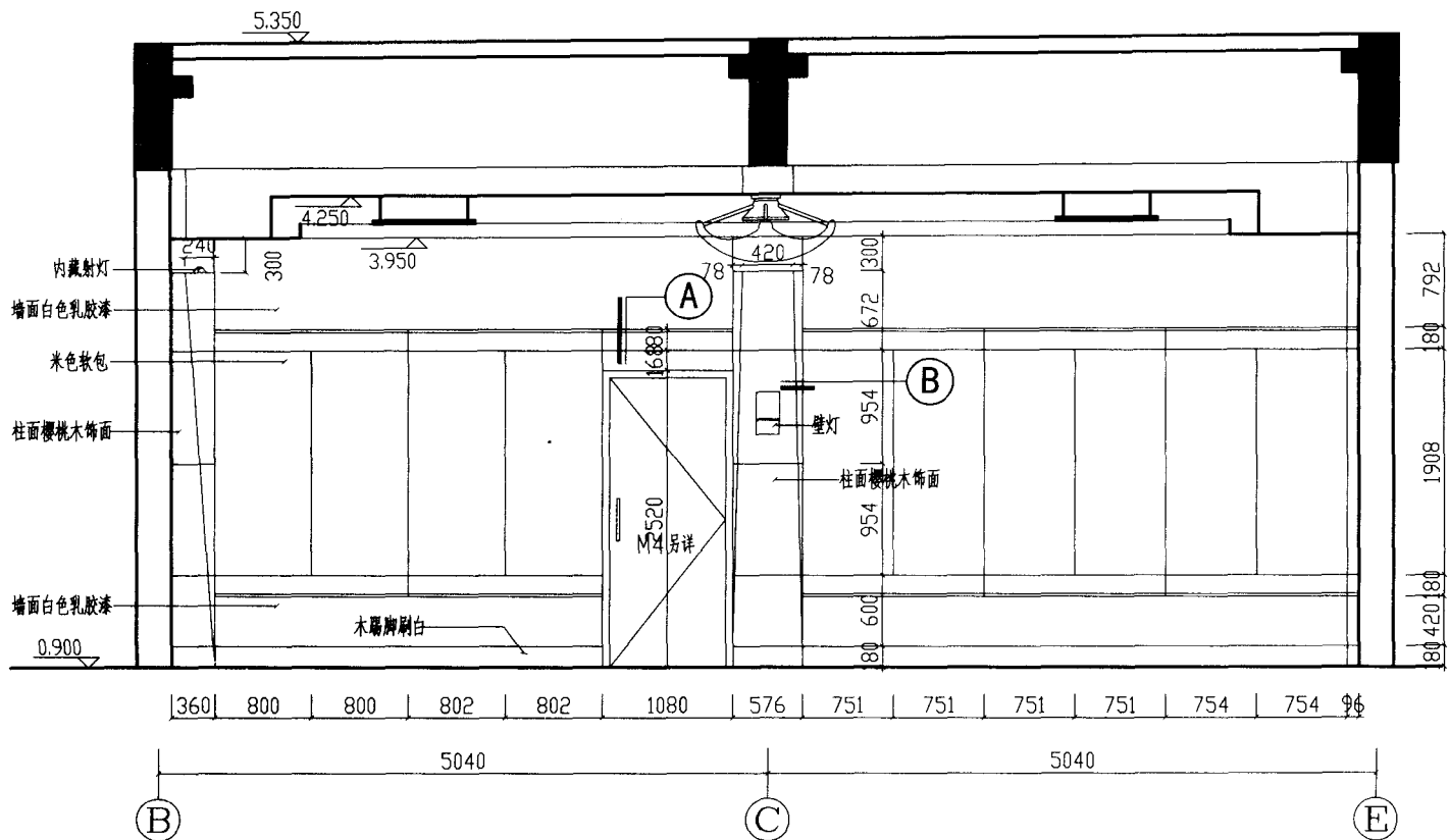
① 贵宾接待室立面图
