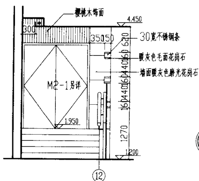
7 前厅立面图
