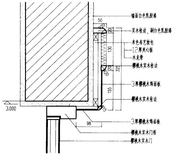
(A) 门套大样图
