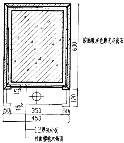
I 柱子大样图
