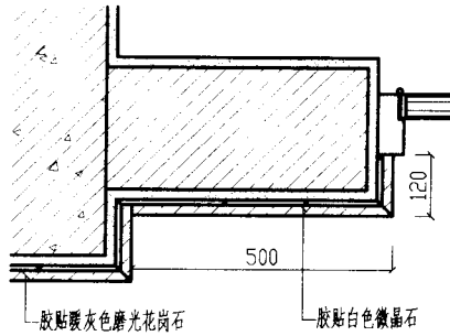
H 墙面大样图
