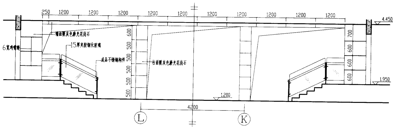
8 前厅立面图
