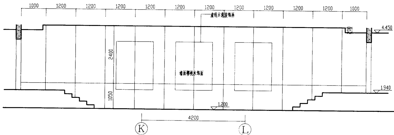
6 前厅立面图
