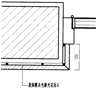
G 墙面大样图
