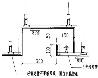
E 吊顶大样图
