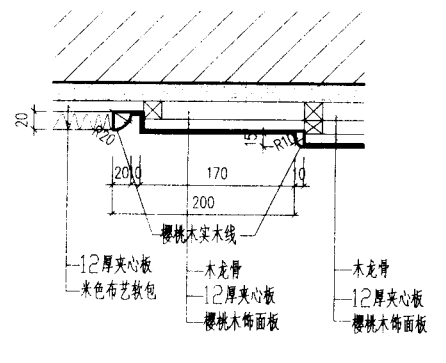
(D) 墙面大样图
