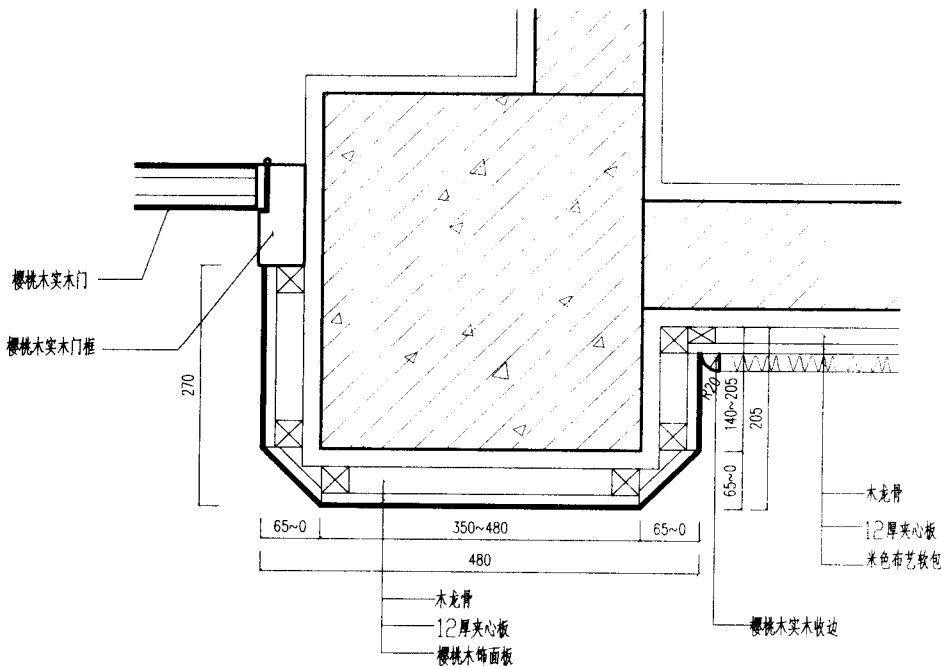
(B) 柱子大样图
