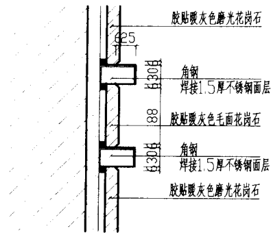
F 墙面大样图
