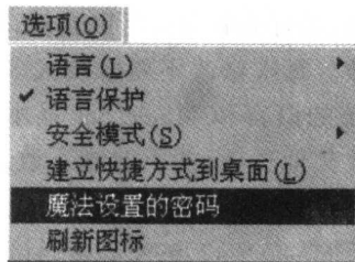
图 1.9 “选项”菜单
